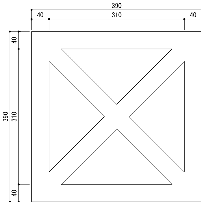
正面図
